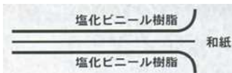
ワーロンシートの構造
